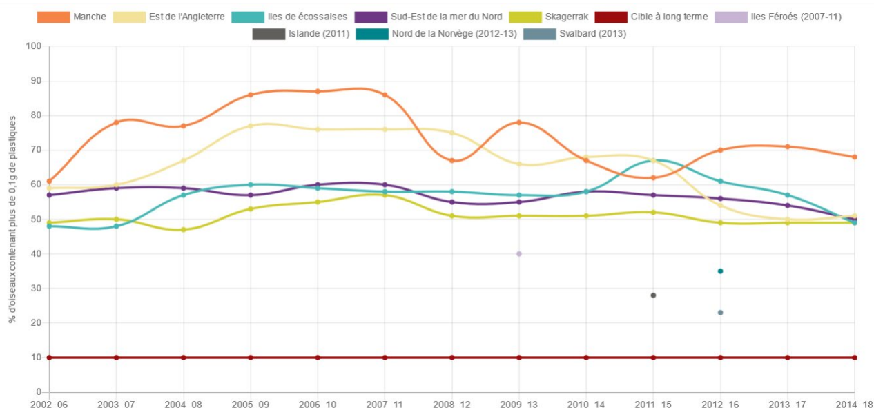
Figure 4. Moyennes glissantes sur cinq ans du pourcentage de fulmars dont l'estomac contient plus de 0,1 g de plastique, depuis 2002. Les données accessoires publiées pour les Iles Féroé, l'Islande, la Norvège septentrionale et le Svalbard sont incluses pour illustrer les niveaux de plastiques ingérés plus faibles plus au Nord de la zone maritime OSPAR, mais qui sont néanmoins bien au-dessus de l'objectif à long terme d'OSPAR. Veuillez noter que ce graphique n'est qu'une aide visuelle, et non une analyse statistique.
